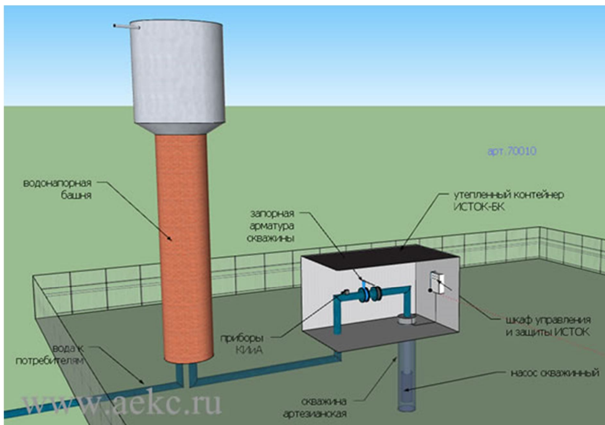
Схема идеального водозаборного узла системы водоснабжения потребителей муниципального образования.
