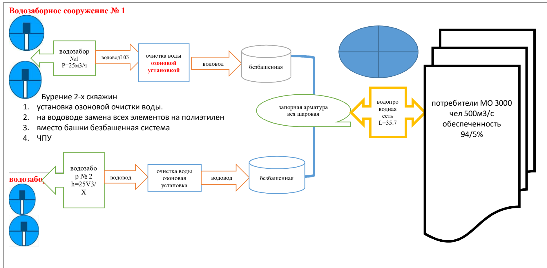
Реконструированная схема водоснабжения муниципального образования «Кошехабльское сельское поселение»
