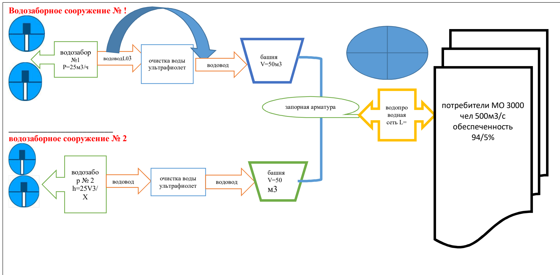
Структурная схема водоснабжения муниципального образования «Кошехабльское сельское поселение»
